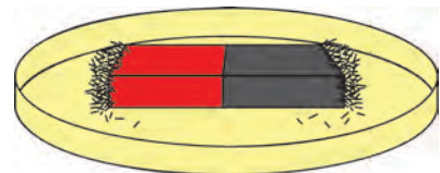
15.7 : Magnetic power
